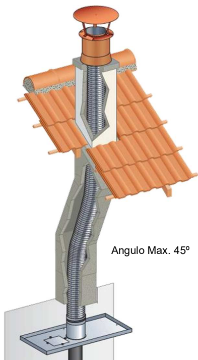
Instalação tipo de Tubo Flexível em Inox
